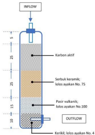
Gambar 1. Model filter air (Sumber: Penulis, 2020)
