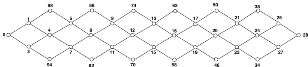
Gambar 2. Graf tali R(6)
