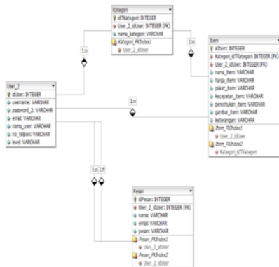
Gambar 11. Relasi Antar Tabel
