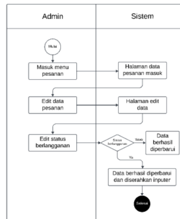
Gambar 9. Skenario Pesanan di Tindak Lanjut Admin
