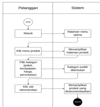
Gambar 6. Skenario Pelanggan Cek Rekomendasi
