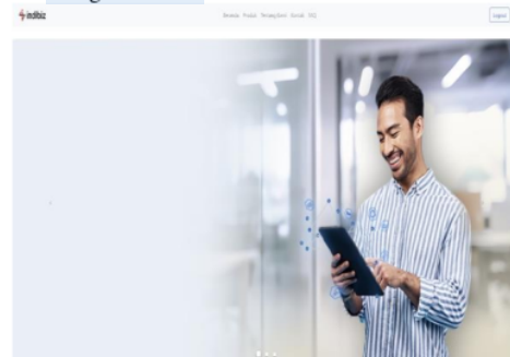
Gambar 12. Halaman Utama
