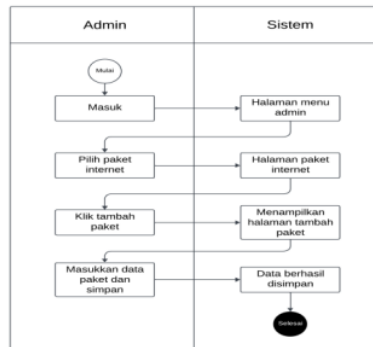
Gambar 5. Skenario Tambah Produk
