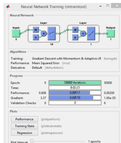
Gambar 4. Training JST Backpropagation pada Matlab
