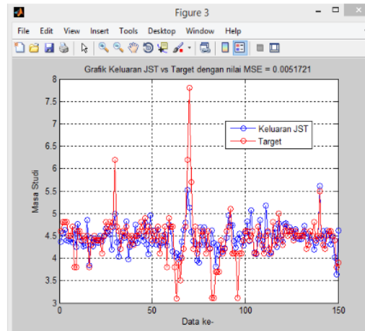
Gambar 3. Hasil Pelatihan JST Backpropagation
