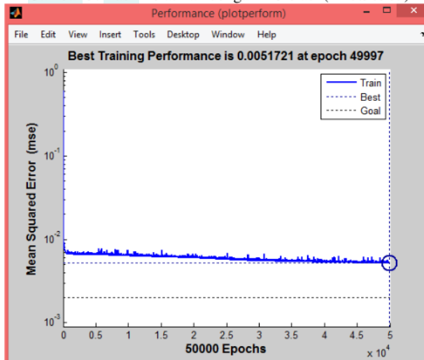
Gambar 6. Grafik Hasil Pelatihan dengan Parameter Epoch 50000
