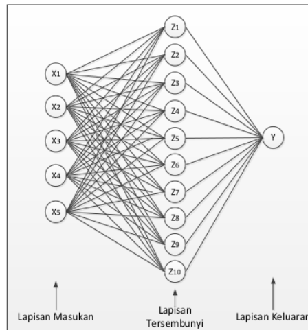
Gambar 1. Arsitektur Jaringan Pengukuran Tingkat Korelasi
