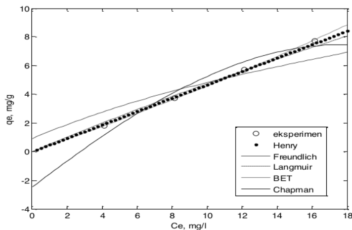
Gambar 1. Kesetimbangan Ion Chrom VI dalam Zeolit pada Berbagai Model
