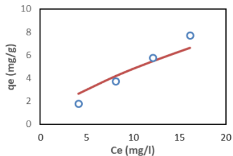
Gambar 3. Kesetimbangan Ion Chrom VI dalam Zeolit pada Model Freundlich
