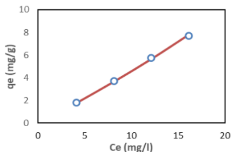
Gambar 5. Kesetimbangan Ion Chrom VI dalam Zeolit pada Model BET
