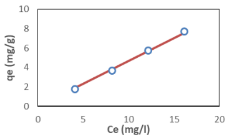
Gambar 2. Kesetimbangan Ion Chrom VI dalam Zeolit pada Model Henry
