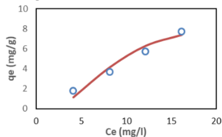
Gambar 6. Kesetimbangan Ion Chrom VI dalam Zeolit pada Model Chapman
