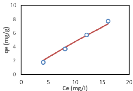
Gambar 4. Kesetimbangan Ion Chrom VI dalam Zeolit pada Model Langmuir
