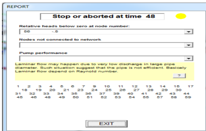
Gambar 2. Jaringan Eksisting setelah di Running
