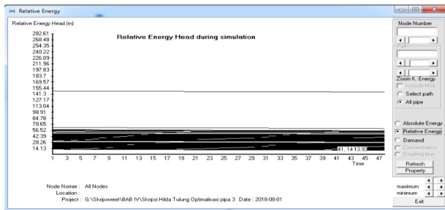
Gambar 4. Tekanan relatif untuk semua node
