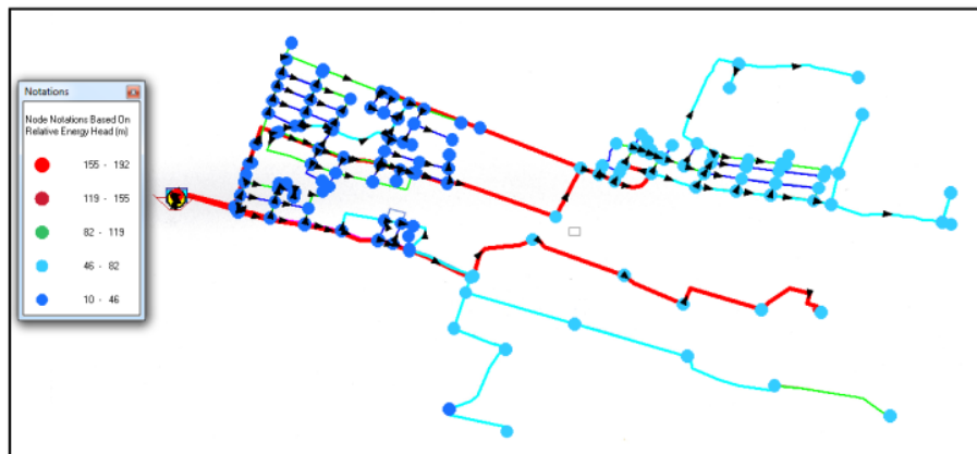
Gambar 5. Kondisi sistem jaringan setelah optimalisasi
