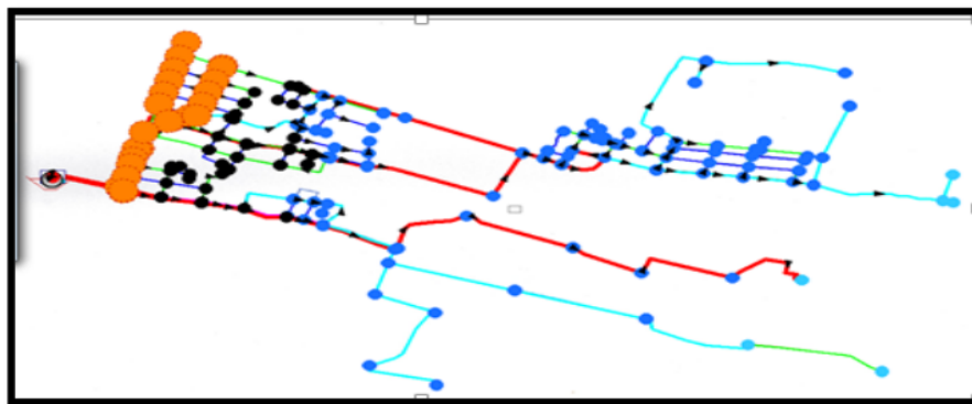
Gambar 1. Jaringan Pipa Eksisting Wilayah Tulung
