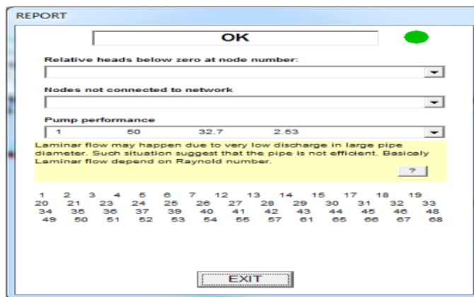
Gambar 3. Laporan hasil simulasi optimalisasi
