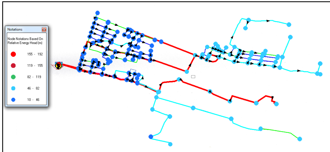
Gambar 5. Kondisi sistem jaringan setelah optimalisasi
