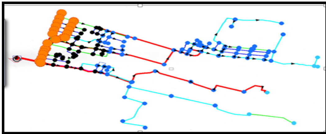
Gambar 1. Jaringan Pipa Eksisting Wilayah Tulung
