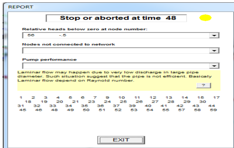
Gambar 2. Jaringan Eksisting setelah di Running
