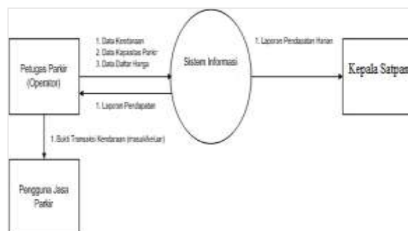
Gambar 2. Diagram Konteks Sistem
