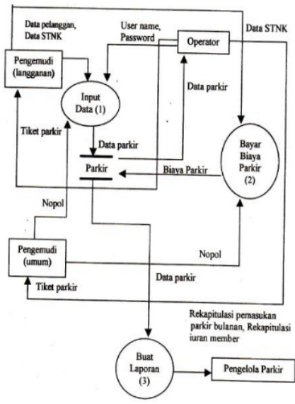
Gambar 2. DFD Level 1
