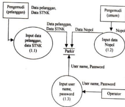
Gambar 3. DFD Level 2
